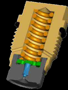
Valvula limitadora De alta pressão
